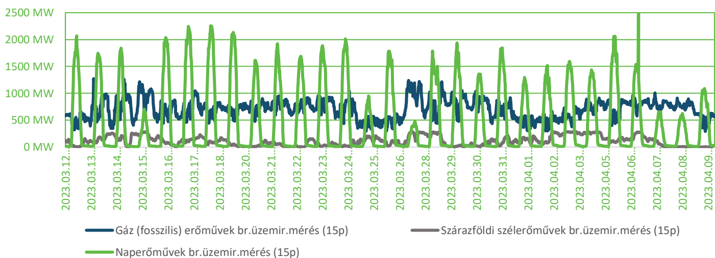
Egyes hazai erőművek villamostermelése (MW), elmúlt 30 nap (Forrás)
